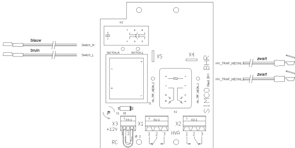
Abbildung 10: Optionale BHR-Leiterplatte
