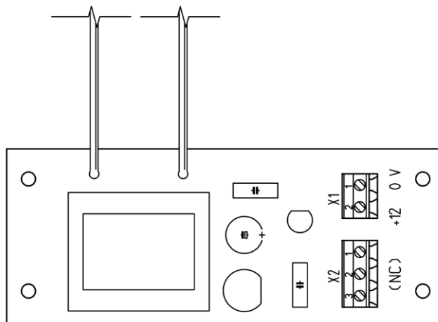
Abbildung 12: Optionale M-Leiterplatte
