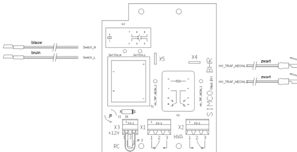
Afbeelding 10: optieprint BHR
