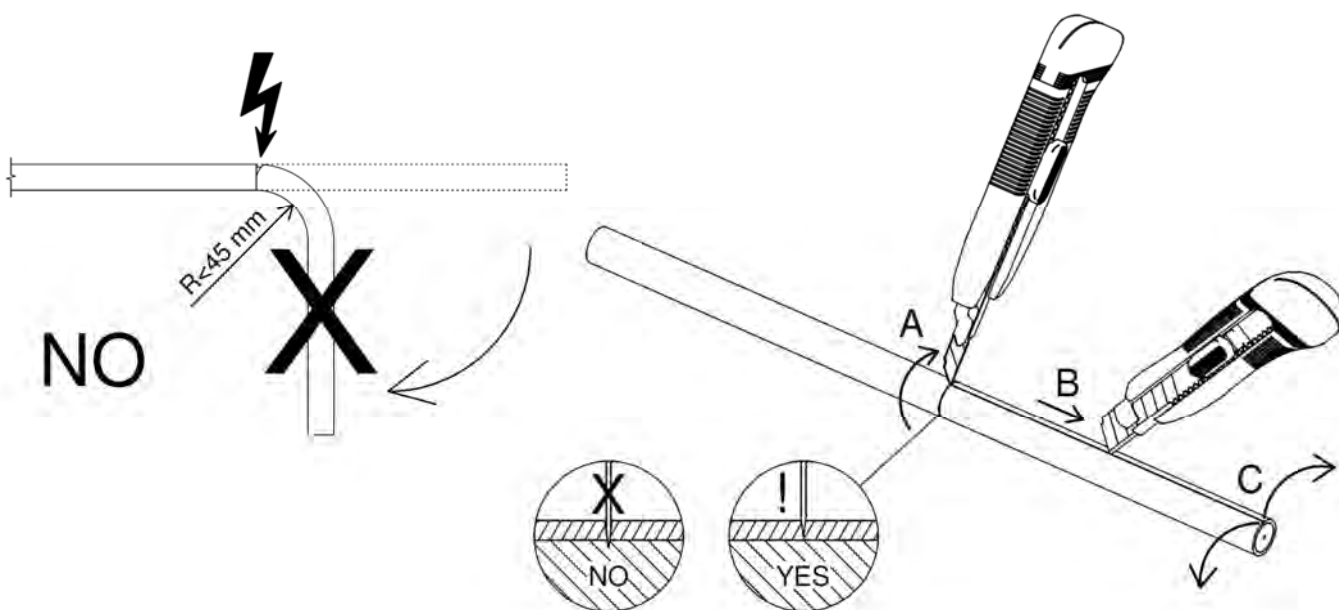
Afbeelding 5: kabelmantel strippen
